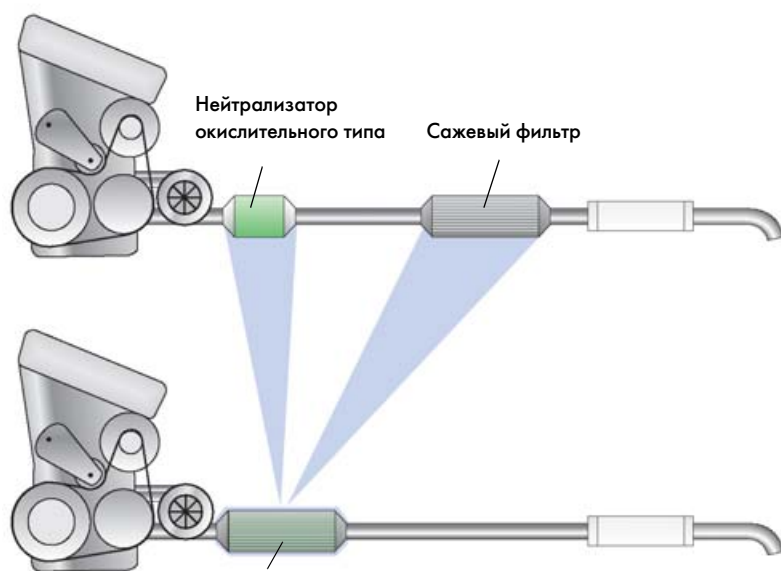
Сажевый фильтр с каталитическим покрытием
