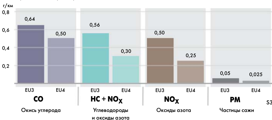
Предельные выбросы вредных веществ автомобилей с дизелями
