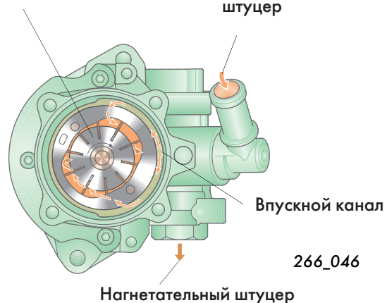
Впускной штуцер
