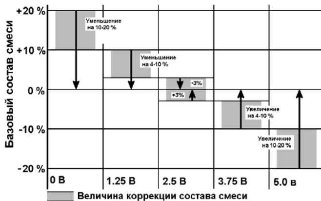
Рис. 4. Коррекция состава топливной смеси.
