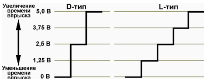
Рис. 9. Коррекция состава смеси по напряжению Vf
