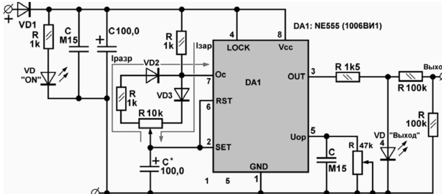
Рис. 10. Схема имитатора кислородного датчика.
