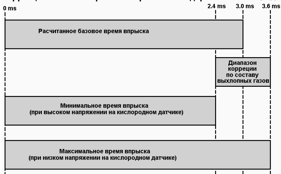
Рис. 2. Коррекция базового времени впрыска по содержанию кислорода.
